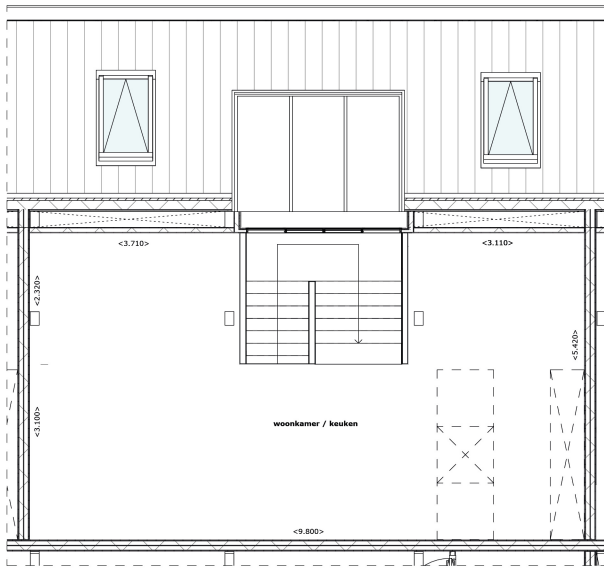
Plattegrond verdieping 04 1:50
